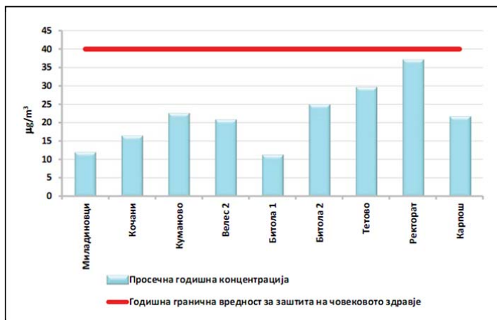
Слика бр. 18 Просечните годишни концентрации на \text{NO}_2 во воздухот
